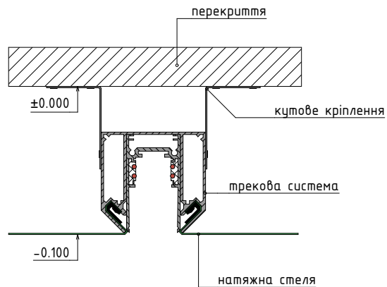
Схема монтажу трекової системи та натяжної стелі
